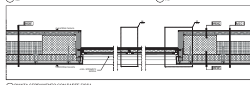
04 PIANTE SERRAMENTO CON PARTE FISSA
