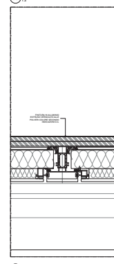
07 NODO ORIZ. CENTRALE
