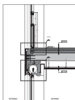
02 SEZIONE SERRAMENTO CON PARTE FISSA
