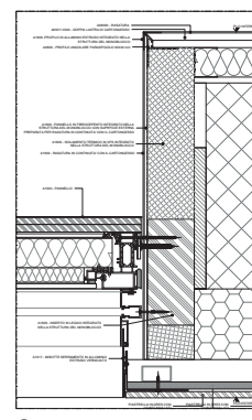
08 NODO ORIZ. LATERALE
