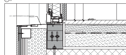
06 NODO VERTICALE INFERIORE
